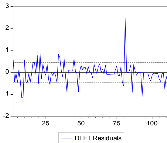
Figure 5 – Résidus du modèle ARIMA(0,1,1)
